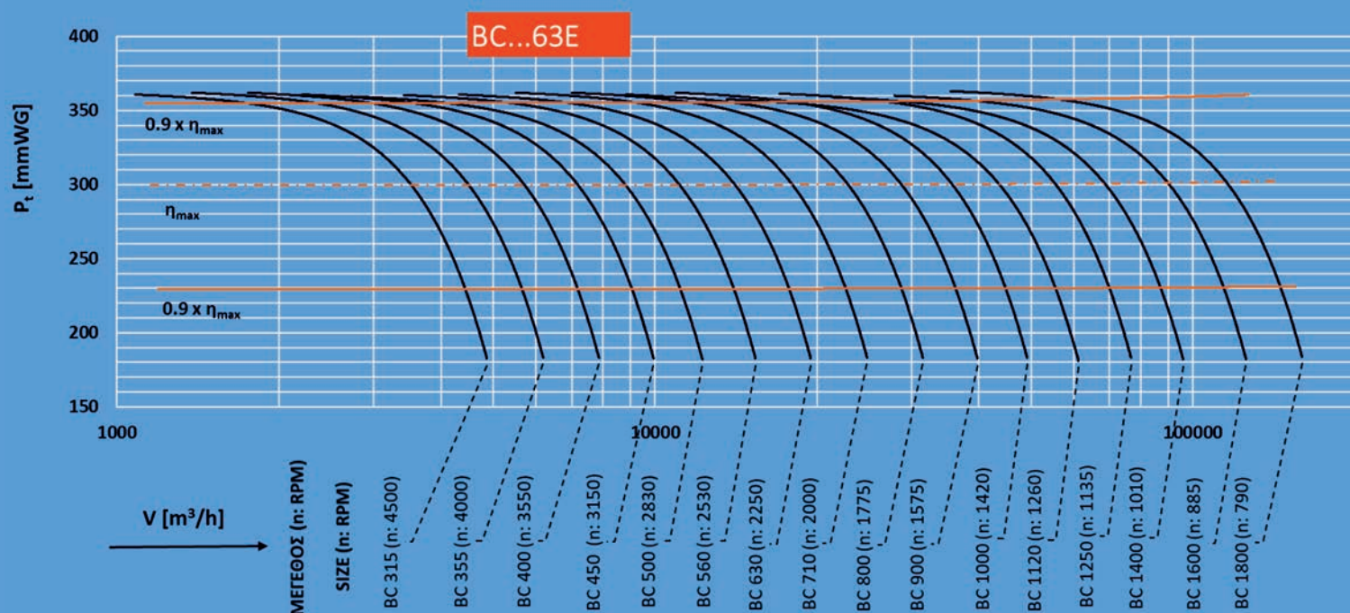
Chart 1: BC...63E Series Performance Curves | Διάγραμμα 1: Καμπύλες Απόδοσης Σειράς BC...63E
