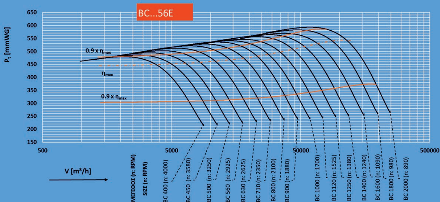
Chart 1: BC...56E Series Performance Curves | Διάγραμμα 1: Καμπύλες Απόδοσης Σειράς BC...56E
