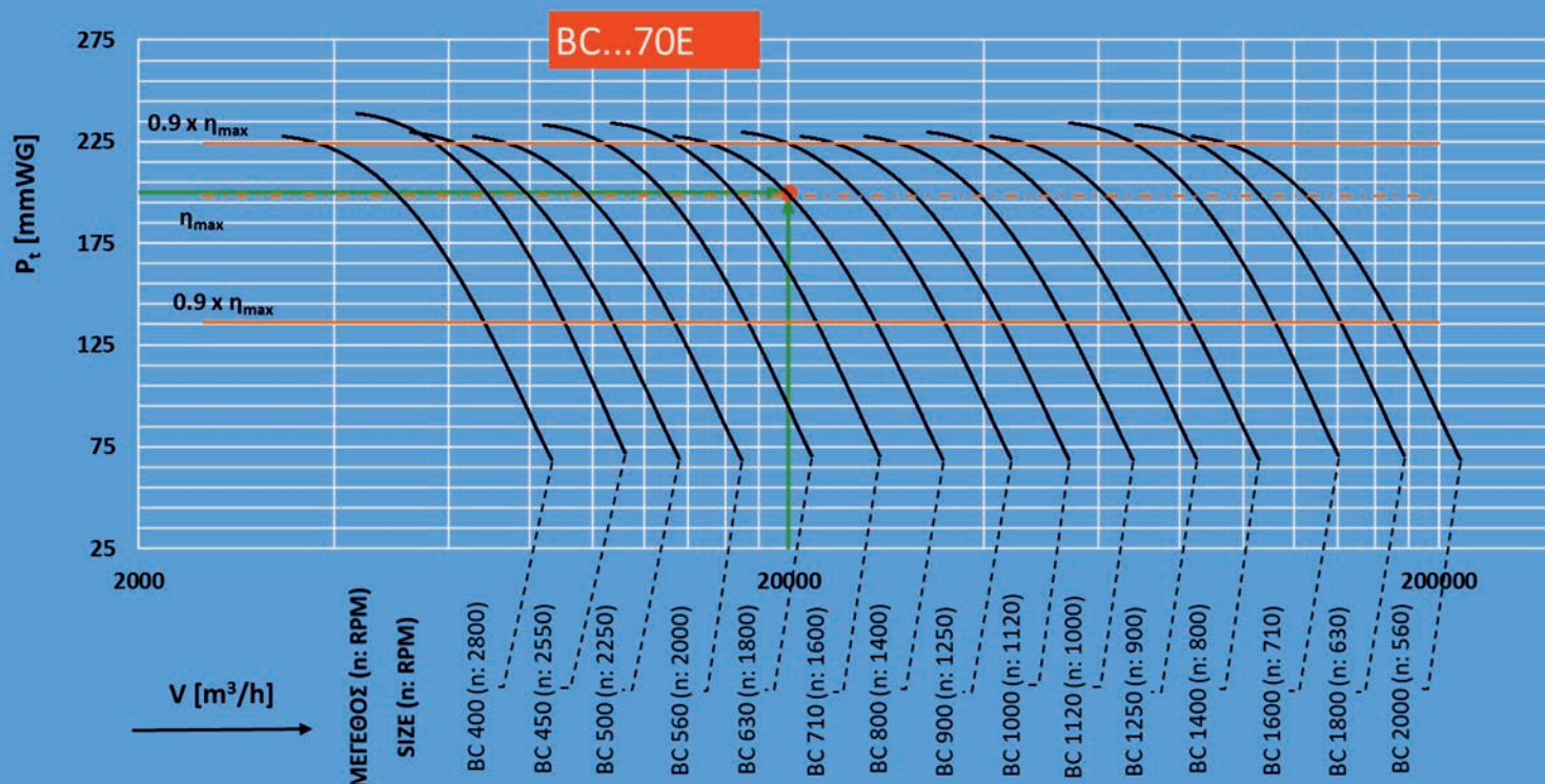
Chart 1: BC...70E Series Performance Curves | Διάγραμμα 1: Καμπύλες Απόδοσης Σειράς BC...70E
